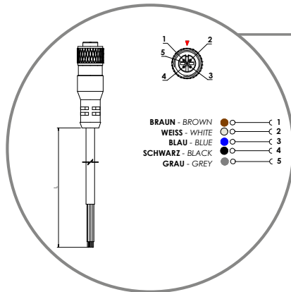
cod. CBL200-001 2 m Kabel mit M12-Verbinder 2 mt cable with connector M12
